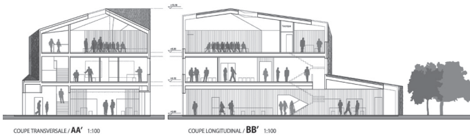
COUPE TRANSVERSALE / AA' 1:100
